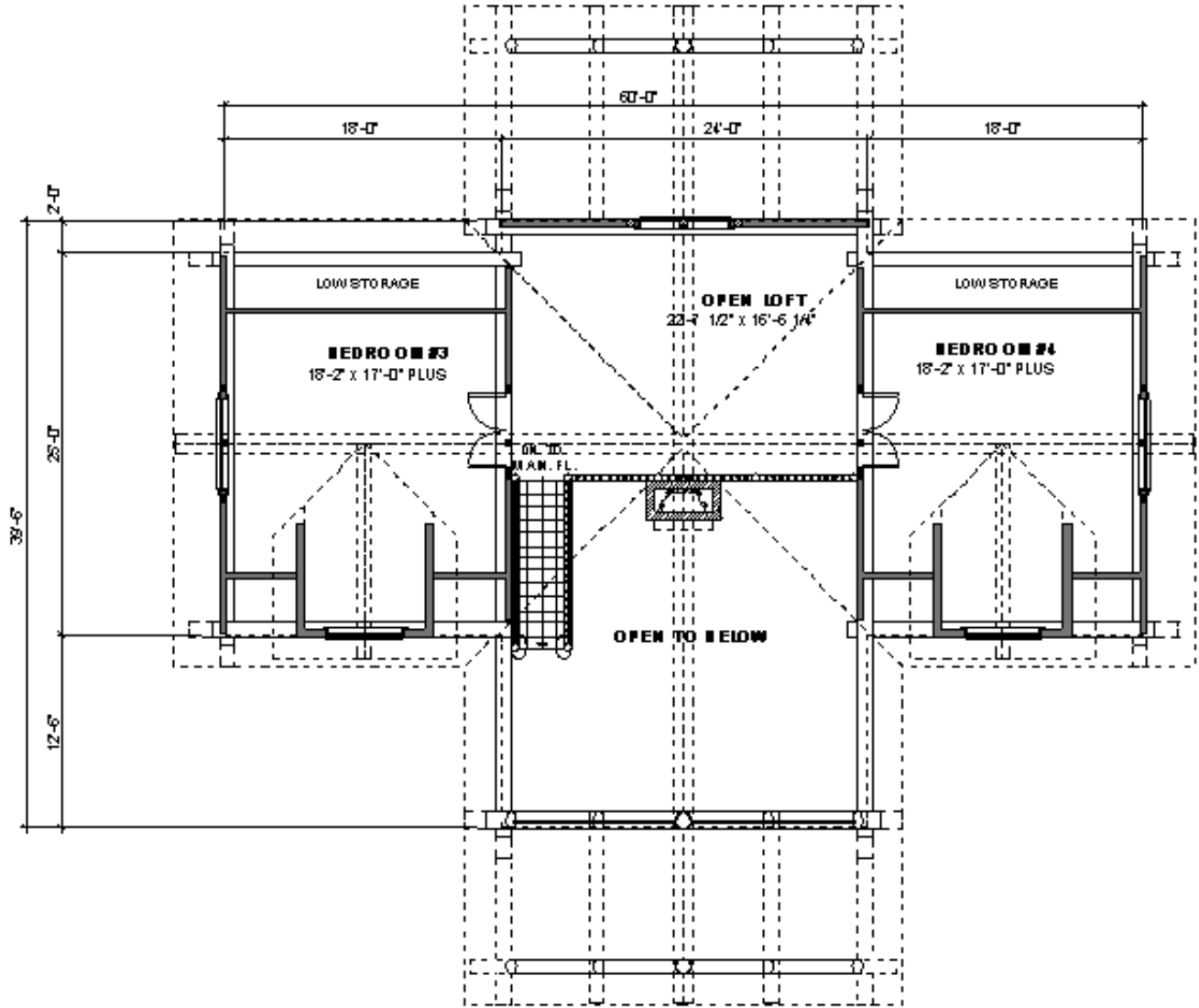
LOFT FLOOR PLAN 1,308 S.Q.F.T.
